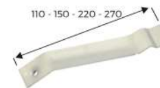
Patte de scellement pour coulisse avec fileté 6MA
