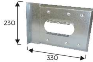
Plaque fixe profondeur 30mm
